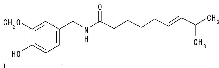
カプサイシンの化学構造
