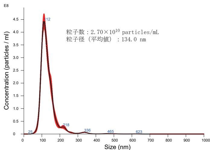
図 2. Nanosight による Leuconostoc mesenteroides 180720-12-1 株由来 EVs の粒度分布測定例
