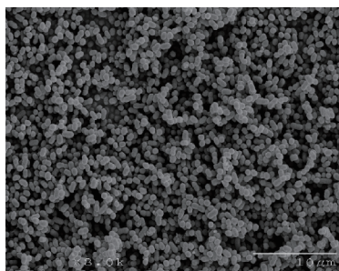
図 1. Leuconostoc mesenteroides 180720-12-1 株の電子顕微鏡画像
