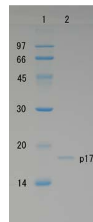
図 1 ポリアクリルアミドゲルによる HIV-1 p17 タンパク質の電気泳動
