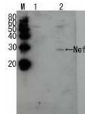
図1 HIV-1 Nef 体を用いたウエスタンブロット法による Nef 原の検出
