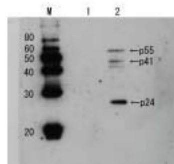
図1 HIV-1 p24 体を用いたウエスタンブロット法による p24 原の検出
